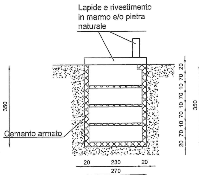
SEZIONE B-B
