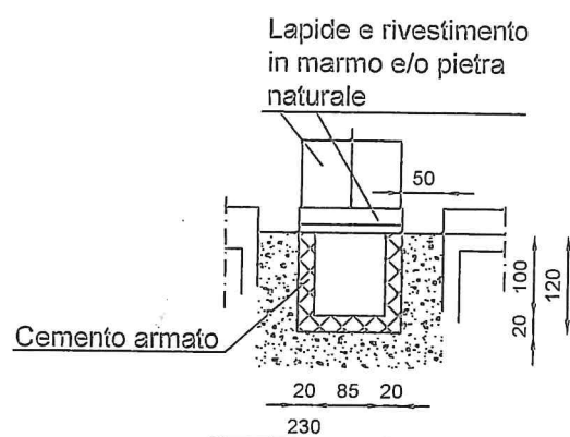
SEZIONE A-A
