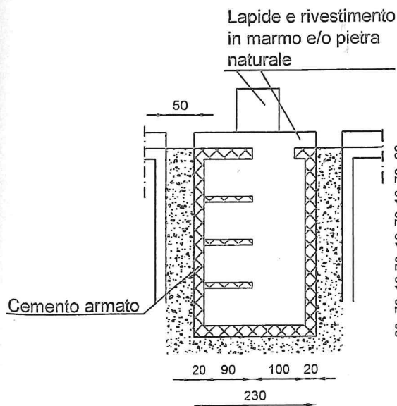
SEZIONE A-A
